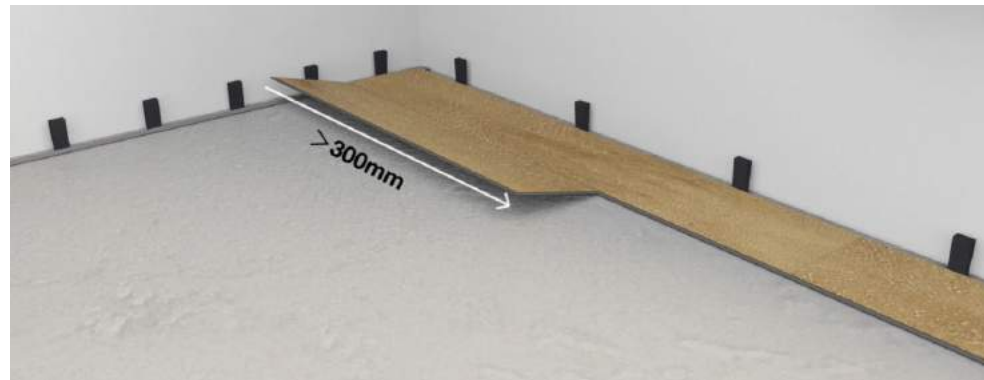
Segunda fila, primer tablón: Comience la segunda fila con la parte cortada del último tablón de la fila anterior. Este pieza debe medir al menos 300 mm / 12". / Second row, first plank: Start the second row with the cut part of the plank of the previous row. This small plank should measure at least 300 mm/12".
