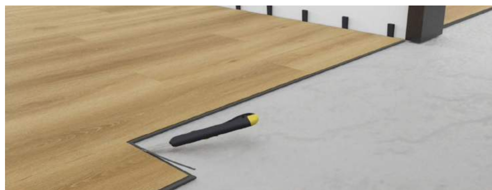
Corte el borde de las ranuras de las tablas adyacentes. / Cut off the lip on the groove of the adjacent planks.
